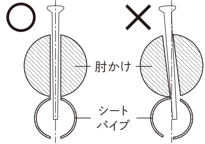
ネジ穴断面イメージ
